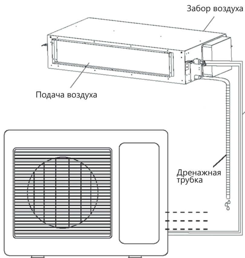
Внутренний блок (типоразмер 18/24/36)
