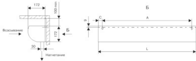
Рис.1. Габаритные и установочные размеры
