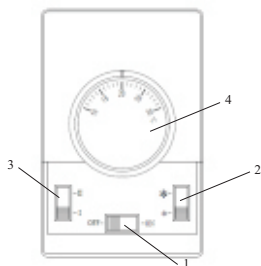
Рис. 1. Пульт управления
